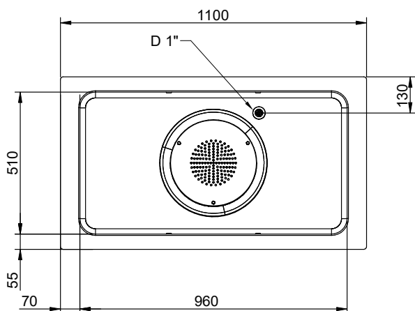
Boven aanzicht
